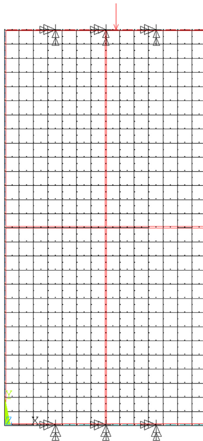
Fig. 27. FEM model.
